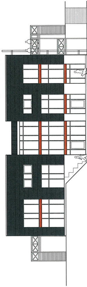
Facade mod nord, mål 1:100
